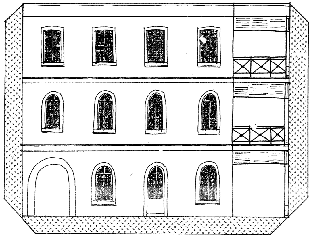
FACADE DROITE
