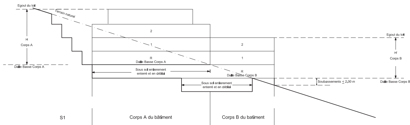
CAS D'UNE CONSTRUCTION EN PLUSIEURS CORPS PENTE MOYENNE DU TERRAIN NATUREL > 25% SOUBASSEMENT < 2,00m
