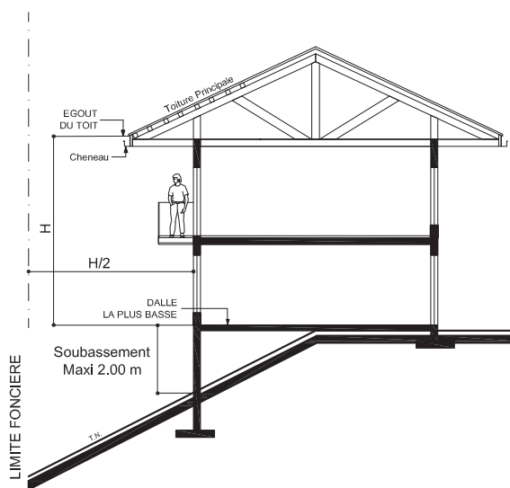
CAS TERRAIN NATUREL EN PENTE > 25% TOITURE CHARPENTÉE AVEC HAUTEUR DE SOUBASSEMENT < 2.00 m
