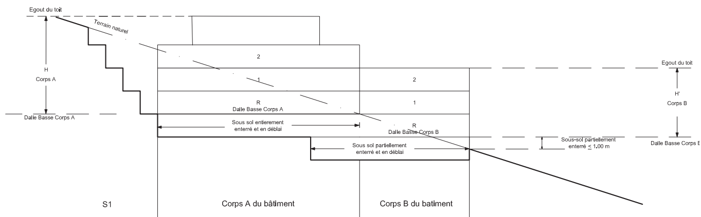
CAS D'UNE CONSTRUCTION EN PLUSIEURS CORPS PENTE MOYENNE DU TERRAIN NATUREL > 25\% SOUS-SOL PARTIELLEMENT ENTERRE
