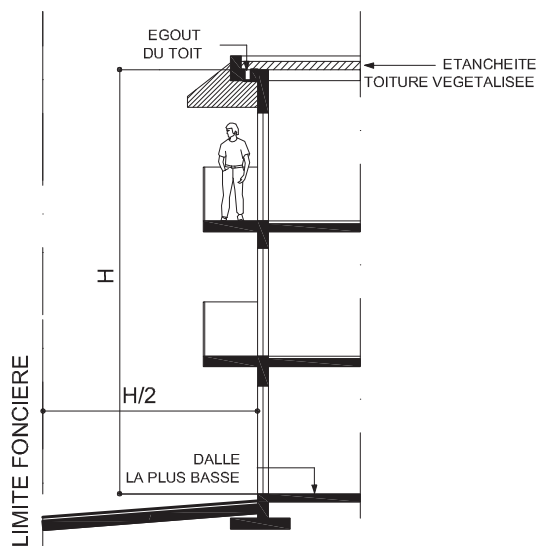
CAS D'UNE TOITURE TERRASSE (VARIANTE)
