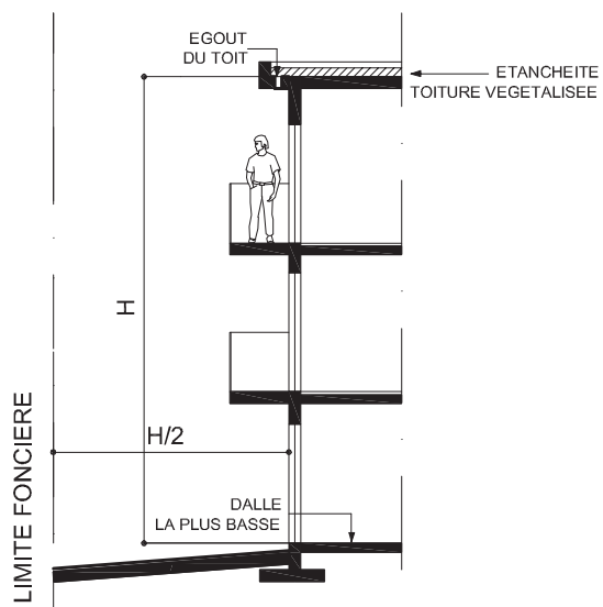
CAS D'UNE TOITURE TERRASSE
