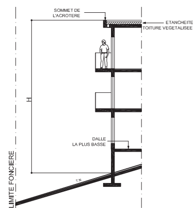
CAS TERRAIN NATUREL EN PENTE < 25% TOITURE TERRASSE AVEC PILOTIS OU SOUBASSEMENT
