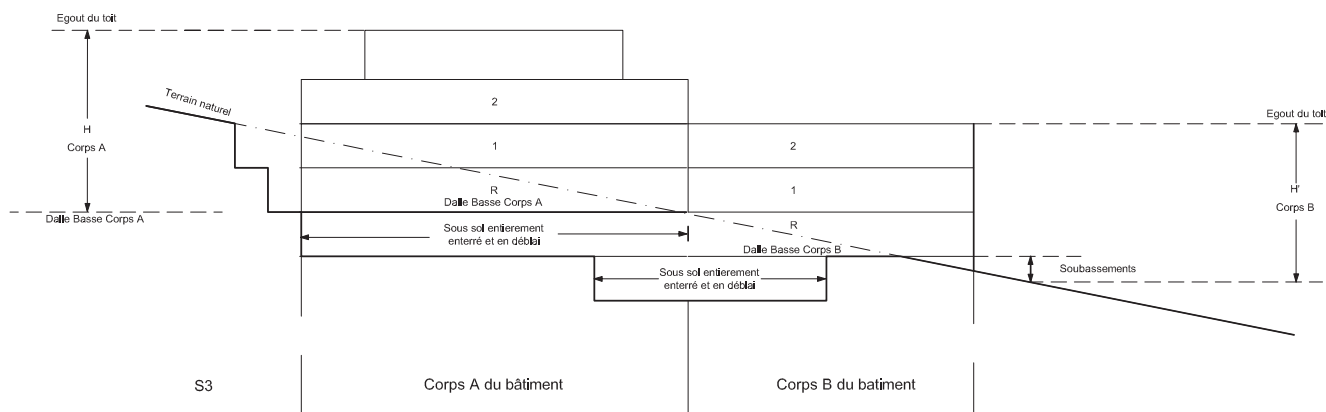
CAS D'UNE CONSTRUCTION EN PLUSIEURS CORPS PENTE MOYENNE DU TERRAIN NATUREL \leq 25\%
