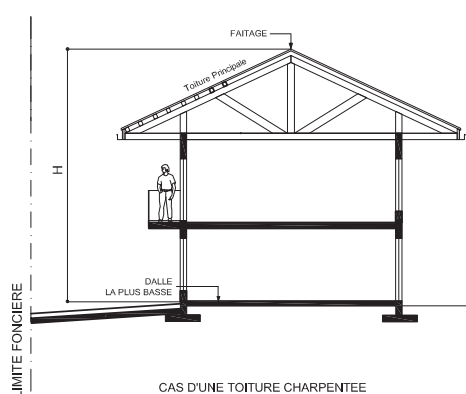
CAS D'UNE TOITURE CHARPENTÉE
