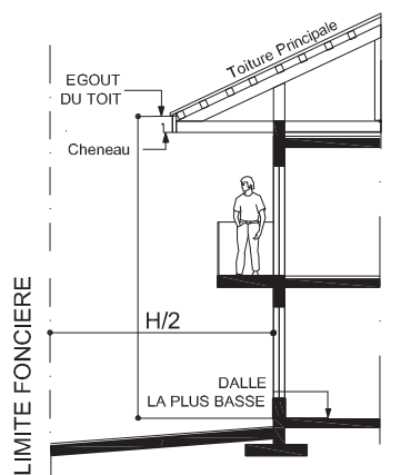
CAS D'UNE TOITURE CHARPENTÉE
