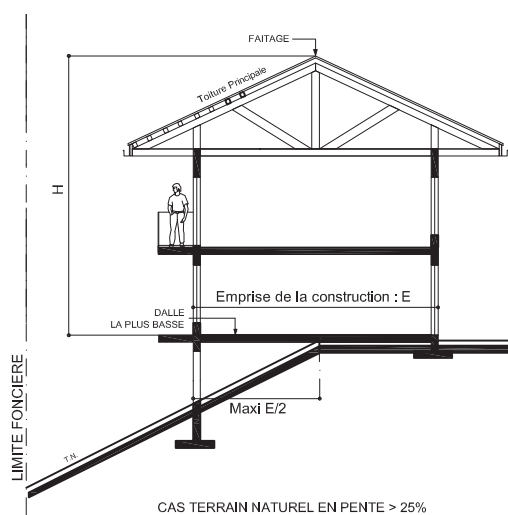
CAS TERRAIN NATUREL EN PENTE > 25% TOITURE CHARPENTEE AVEC PILOTIS PARTIELS
