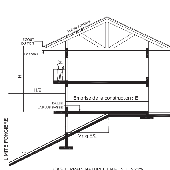
CAS TERRAIN NATUREL EN PENTE > 25% TOITURE CHARPENTÉE AVEC PILOTIS PARTIELS
