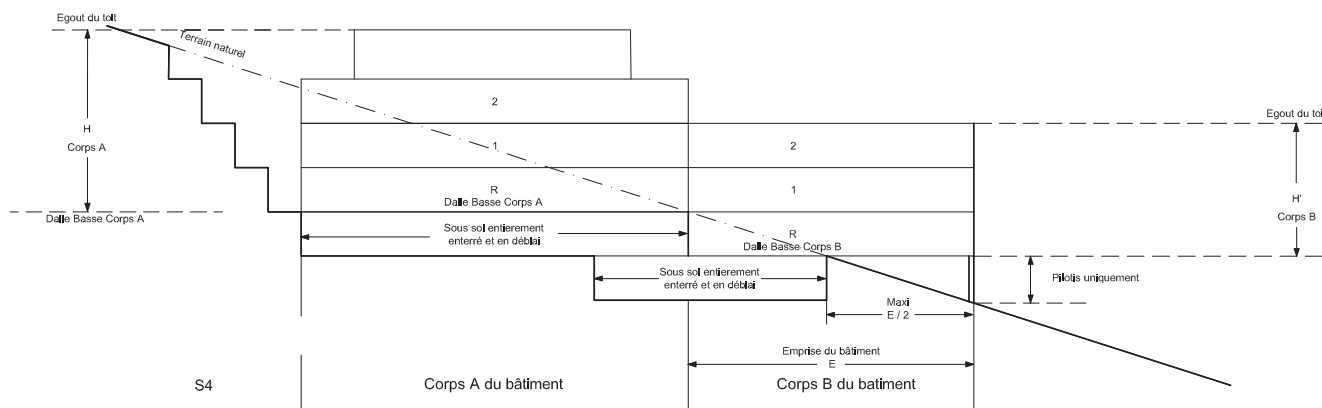
CAS D'UNE CONSTRUCTION EN PLUSIEURS CORPS PENTE MOYENNE DU TERRAIN NATUREL > 25% PILOTIS PARTIELS
