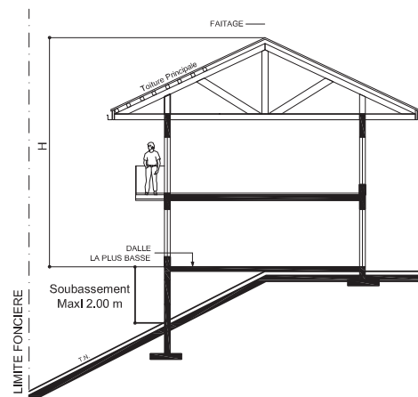
CAS TERRAIN NATUREL EN PENTE > 25% TOITURE CHARPENTEE AVEC HAUTEUR DE SOUBASSEMENT < 2.00 m
