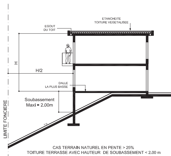
CAS D'UNE TOITURE TERRASSE (VARIANTE)
