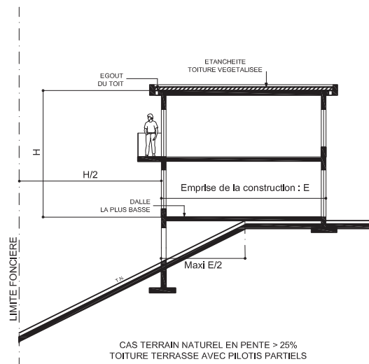
CAS D'UNE TOITURE TERRASSE (VARIANTE)
