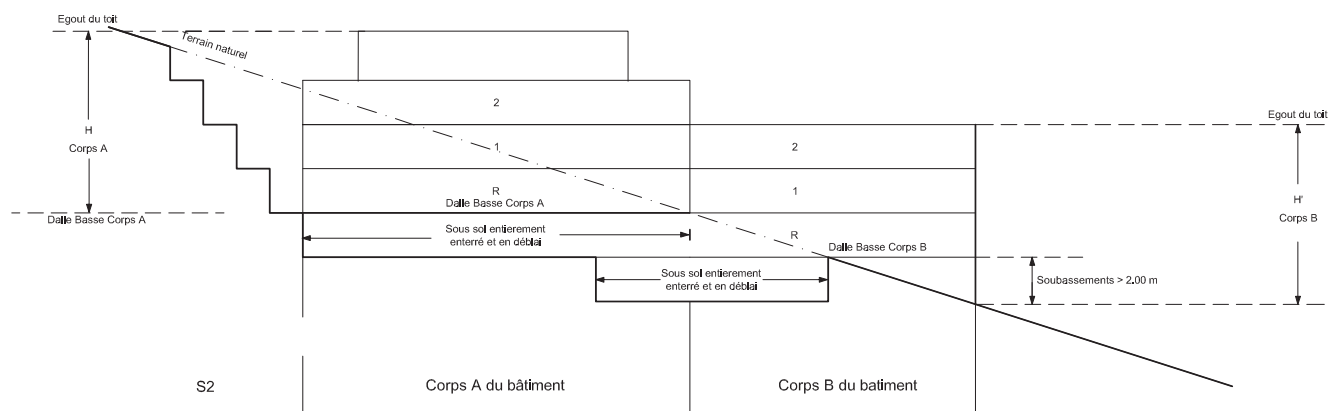
CAS D'UNE CONSTRUCTION EN PLUSIEURS CORPS PENTE MOYENNE DU TERRAIN NATUREL > 25% SOUBASSEMENT > 2,00m
