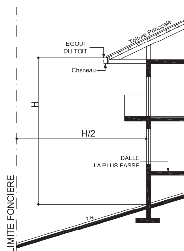
CAS TERRAIN NATUREL EN PENTE < 25% TOITURE CHARPENTÉE AVEC PILOTIS OU SOUBASSEMENT
