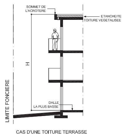
CAS D'UNE TOITURE TERRASSE
