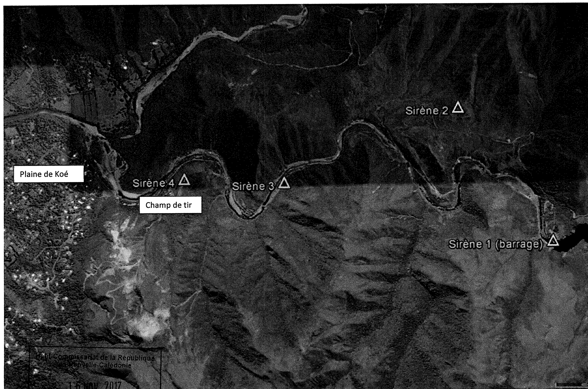
Figure 4 : Implantation des sirènes d'alerte (Triangles jaune).
